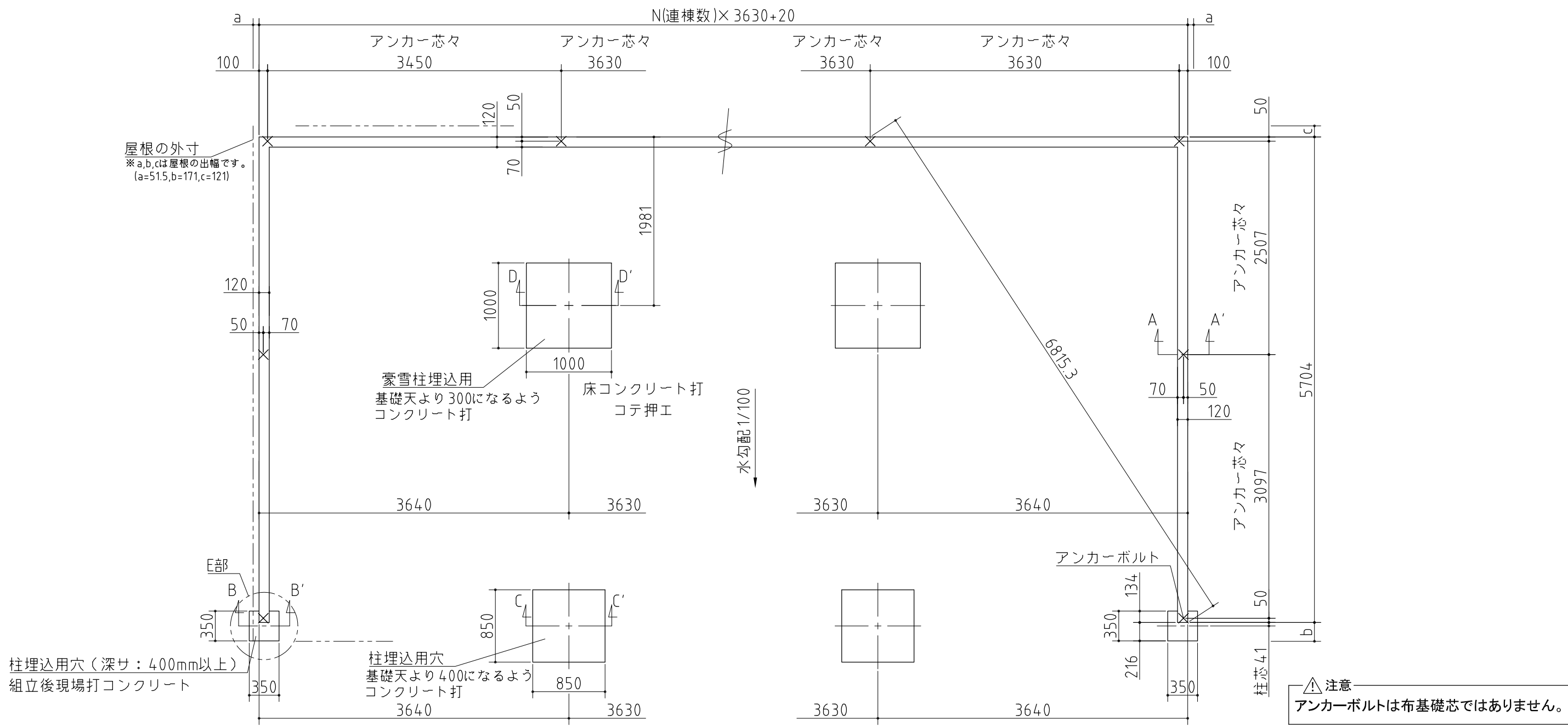
基礎詳細図 S=1/20
